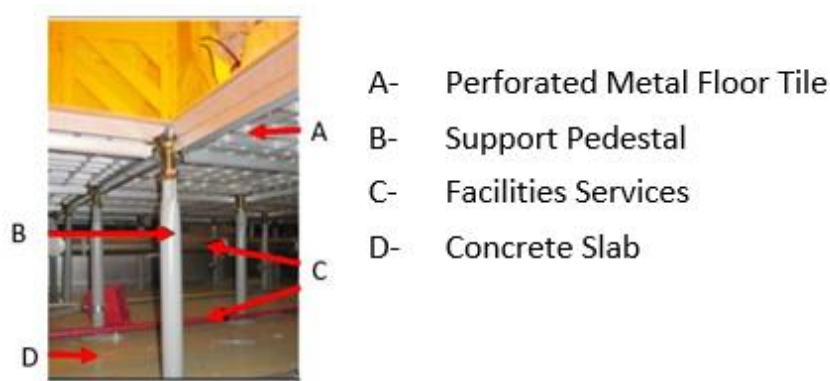
図13 金属製高床の交差するセクション
