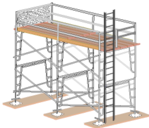
図 28 枠組み足場
